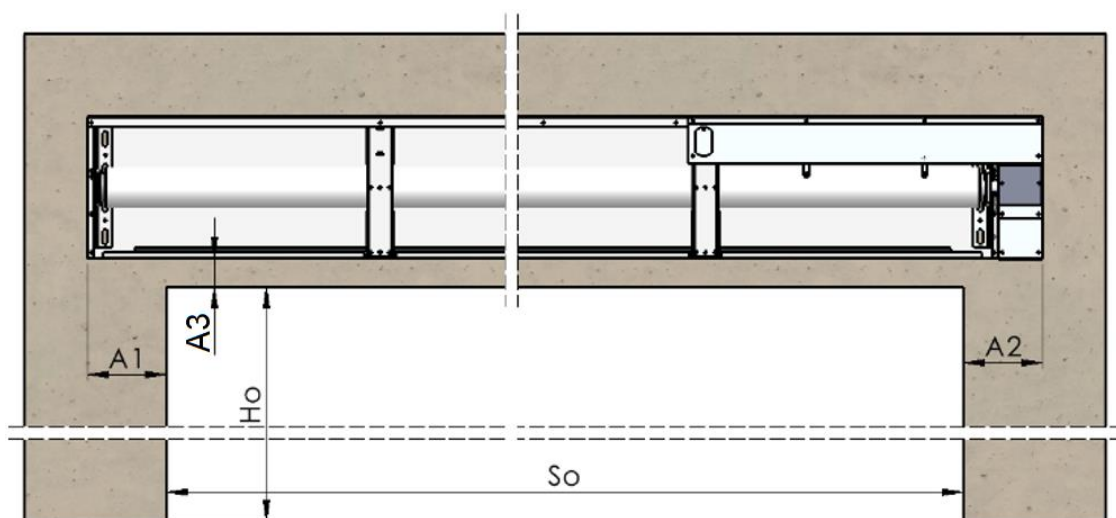
Fig. 4 Emplacement de montage du coffre
