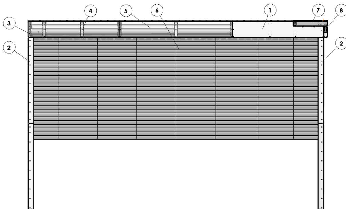
Fig. 2 Vue générale du rideau de feu FIRE DOR FDT
